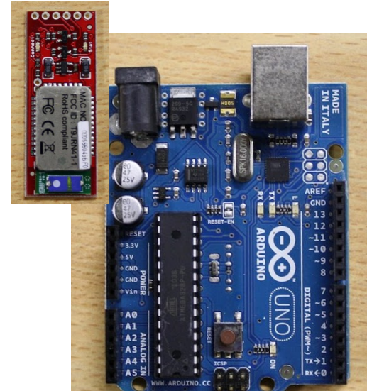
Arduino UNO
