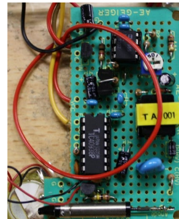
Geiger Counter
